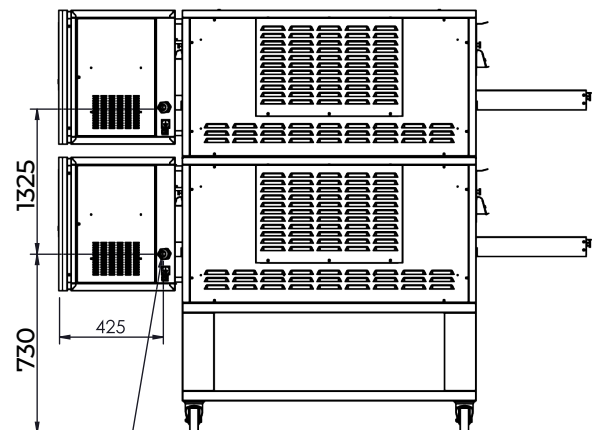
VISTA A
