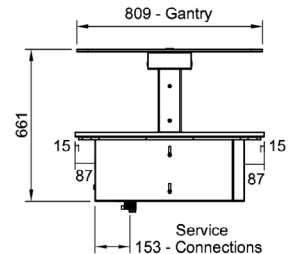
End Elevation
