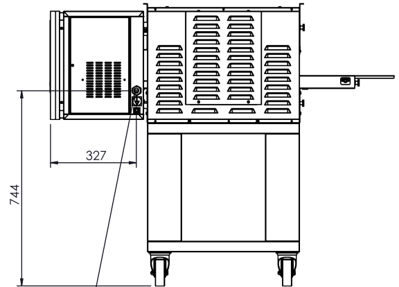
VISTA A
